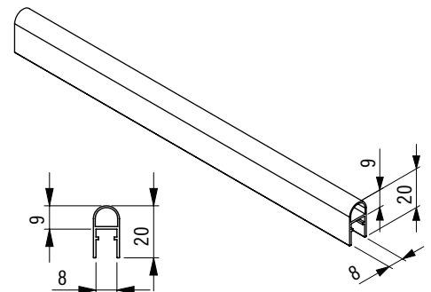
Seal (wall side) 8/42 GXRL0
